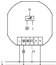
Aansluitvoorbeeld
