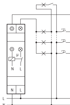
4-draadsschakeling met plafondverlichting, herinschakelbaar
