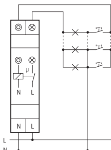
3-draads-schakeling, herinschakelbaar
