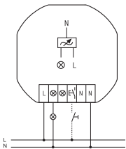
Anslutningsexempel
