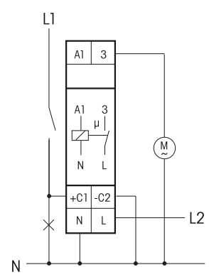
i dörr, ljuset styrs separat Fläktstyrning när fläkt och brytare har olika potentialer
