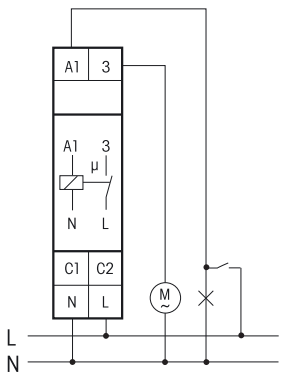
Fläktstyrning via strömställare
