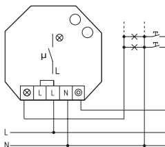
3-draadsaansluiting, herinschakelbaar
