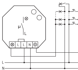
4-draadsaansluiting met zolderverlichting, herinschakelbaar
