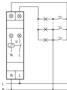
3-draadsaansluiting, herinschakelbaar
