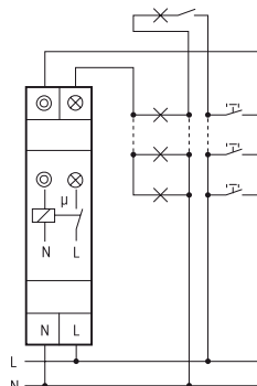
4-draadsaansluiting met zolderverlichting, herinschakelbaar
