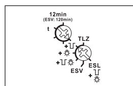
4-draads aansluiting, met zolderverlichting, herinschakelbaar
