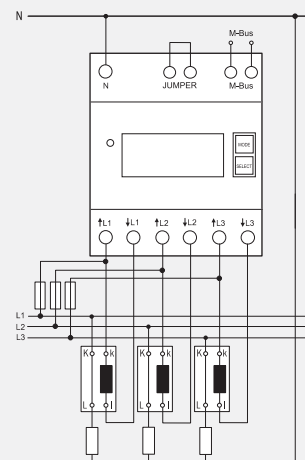
Aansluitvoorbeeld DSZ15WDM-3x5A 4-draads aansluiting 3x230/400V
