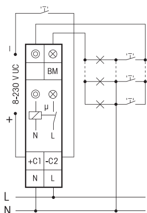
3-draads aansluiting, herinschakelbaar
