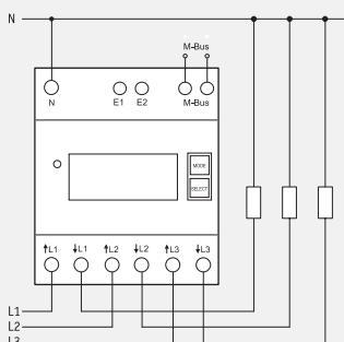
KytKentäesimerkki DSZ15DM-3x80A
