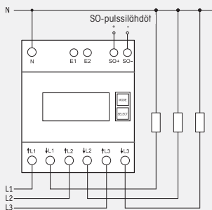
KytKentäesimerkki DSZ12E-3x80A
