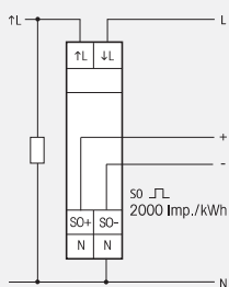
KytKentäesimerkki WSZ15D-32A ja WSZ15DE-32A
