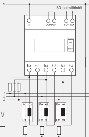
KytKentäesimerkki DSZ15WD-3x5A
