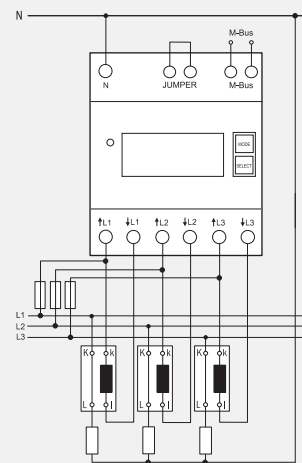
KytKentäesimerkki DSZ15WDM-3x5A
