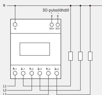
KytKentäesimerkki DSZ12E-3x80A
