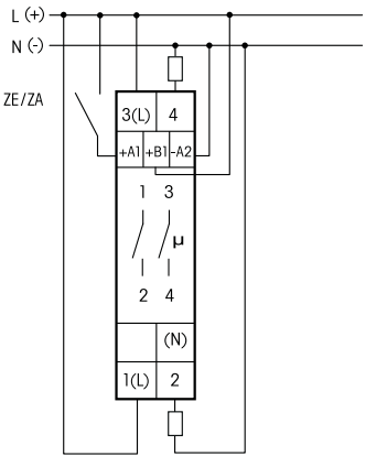
ilman nollapistekytkentää
