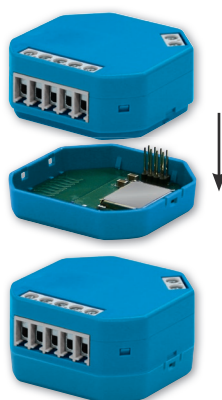
Serie 64-IPM con adaptador EnOcean EOA64
