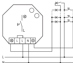
Conexión con 4 hilos, prolongable.
