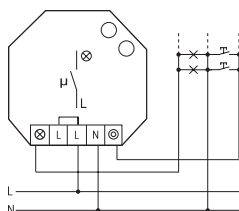
Conexión con 3 hilos, prolongable.
