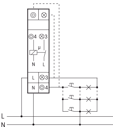
Conexión con 3 cables, prolongable
