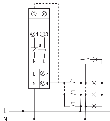
Conexión con 4 cables, prolongable
