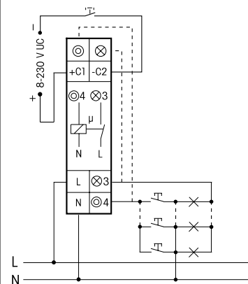
Conexión con 3 cables, prolongable
