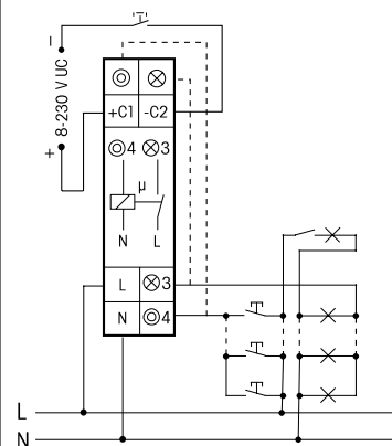
Conexión con 4 cables, prolongable
