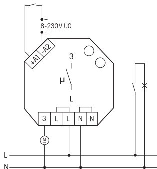
Control de un extractor con tensión pequeña sobre un contacto en la porta
