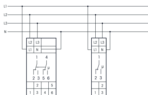
NR12-002-3x230V
