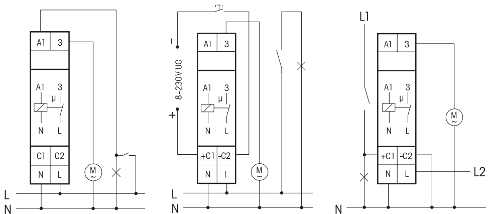
Ventilatorsteuerung über Lichtschalter
