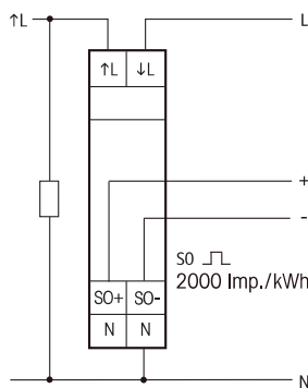
Anschlussbeispiel
