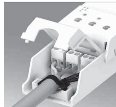
Kabel-Zugentlastung mit handelsüblichen Kabelbindern bis 3,6mm Breite.
