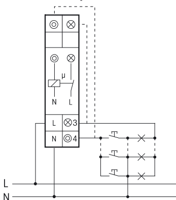
3-Leiter-Schaltung, nachschaltbar.
