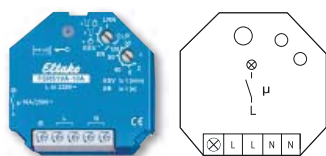
Anschlussbeispiel
