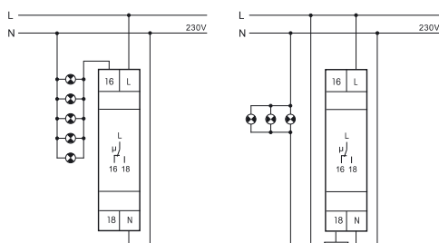
Direkte Ansteuerung der Notleuchten I \leq 16 A Ⓢ Notleuchten mit eigener Akkuvorsorgung Ansteuerung der Notleuchten über Schaltschütz I > 16 A Ⓢ Notleuchten mit eigener Akkuvorsorgung
