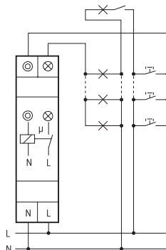
4-ledar system, vindbelysning, med nollställning
