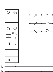
3-ledar system, med nollställning
