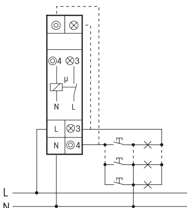
3-draadsaansluiting, herinschakelbaar
