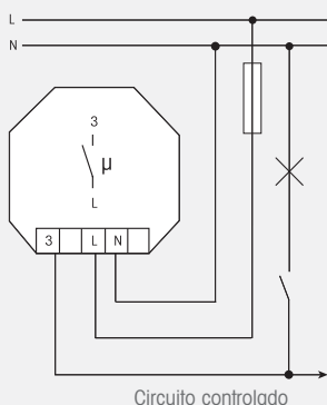
Circuito controlado
