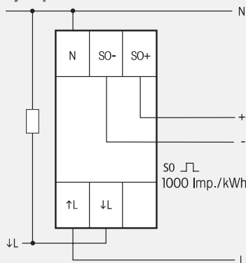
Contador conectado, sin detección de consumo
