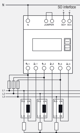
Ejemplo de conexión 3 fases mas N 3x230/400V
