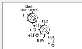
Conexión con 4 hilos, con iluminación del desván, prolongable.
