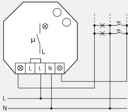
Conexión con 3 hilos, prolongable.
