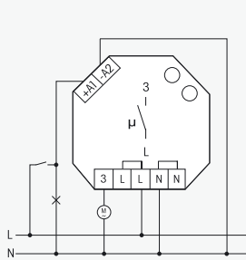
Control de un extractor sobre un interruptor de luz
