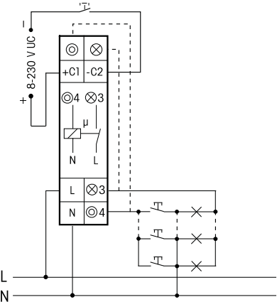
3-Leiter-Schaltung, nachschaltbar.
