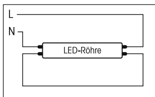
ohne Starterüberbrückung (EVG)
